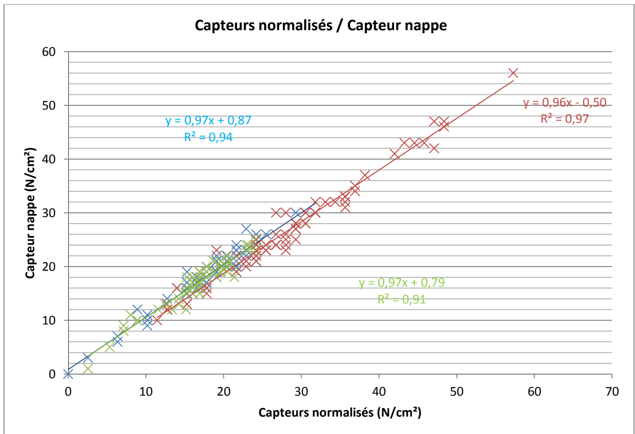
Figure 9 : comparaison des mesures avec les capteurs de force normalisés et celles avec les capteurs de pression de la nappe.
