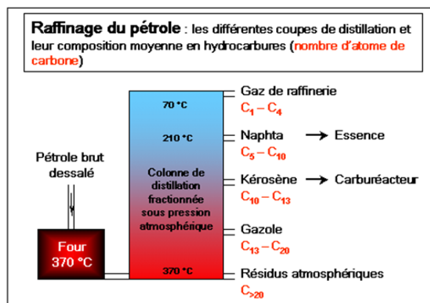
Figure 3 : La distillation atmosphérique
