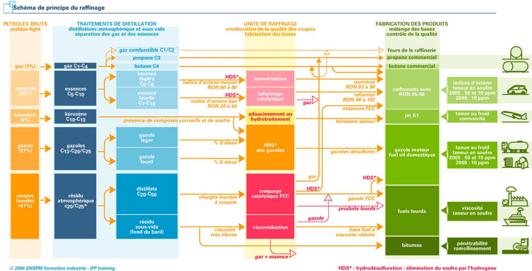
Figure 4 : Schéma de principe du raffinage [47]
